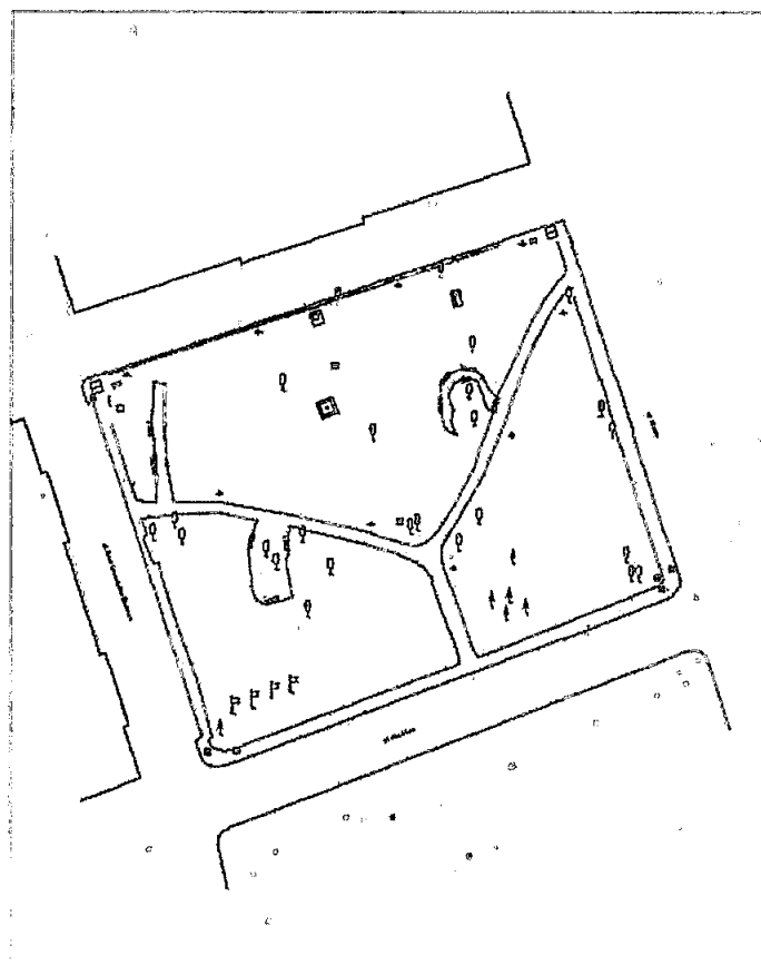
Ažurna geodetska situacija – novo stanje R 1:250
